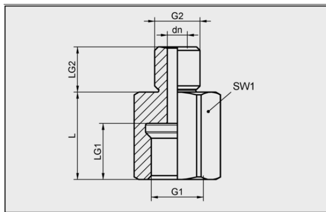
デザインデータ SA-NIP N009 G1/4-IG DN440
