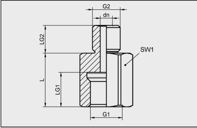
Tasarım verileri SA-NIP N009 G1/4-IG DN440
