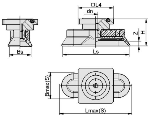
Dati di costruzione SAOG-S 95x40 NBR-60 RA
