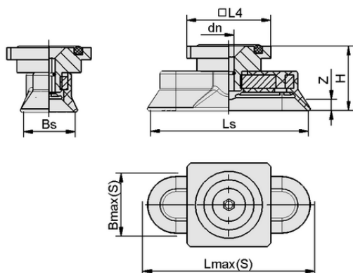
Конструктивные данные SAOG-S 80x30 NBR-60 RA
