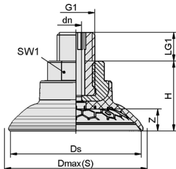
Dati di costruzione SAG 80 NBR-60 G1/4-AG
