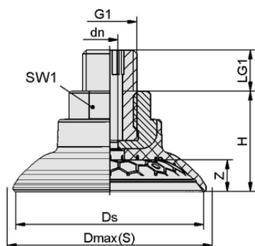
Конструктивные данные SAG 60 NBR-60 G1/4-AG
