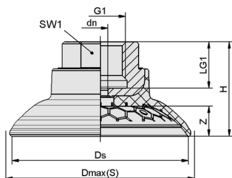
デザインデータ SAG 60 NBR-60 G3/8-IG
