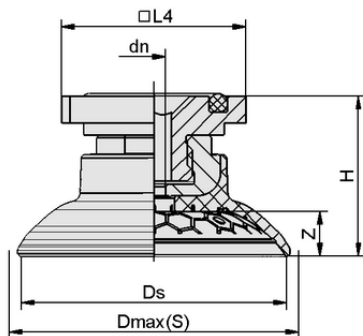
Données de construction SAG 45 NBR-60 RA
