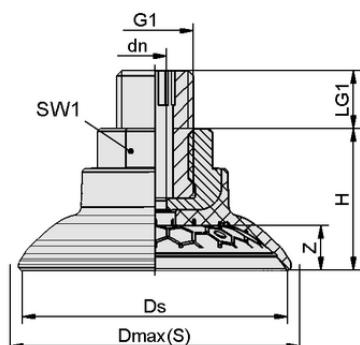
デザインデータ SAG 45 NBR-60 G1/4-AG
