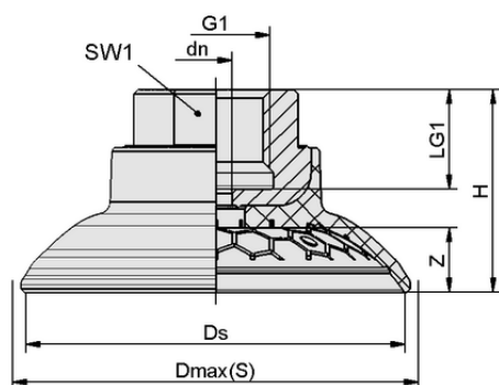
デザインデータ SAG 45 NBR-60 G1/4-IG
