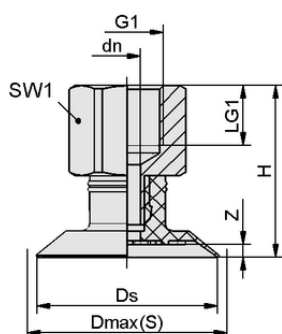
Конструктивные данные SGPN 20 SI-50 G1/8-IG
