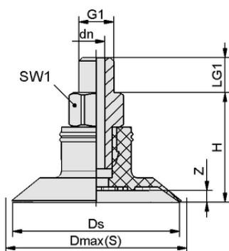
Datos de diseño SGPN 20 NK-40 M5-AG
