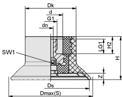
Конструктивные данные SAFT-C 80 NBR-60 M10-AG
