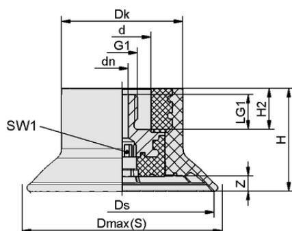
デザインデータ SAFT-C 80 NBR-60 M10-AG
