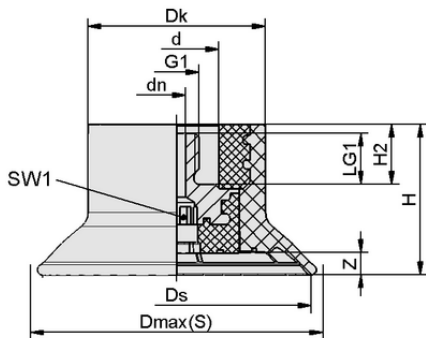
Datos de diseño SAFT-C 60 NBR-60 M10-AG
