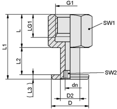
Tasarım verileri SA-NIP N041 G1/4-IG DN440
