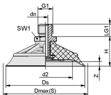
Конструктивные данные SHFN 85 NK-45 G1/4-AG MOS-TV
