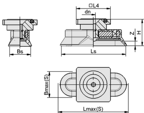
デザインデータ SAOG 60x20 NBR-45 RA
