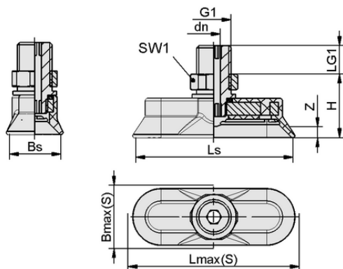
デザインデータ SAOG 60x20 NBR-45 M10-AG
