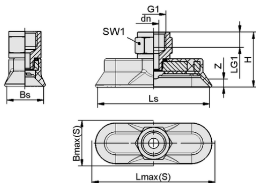
Données de construction SAOG 60x20 NBR-45 G3/8-IG
