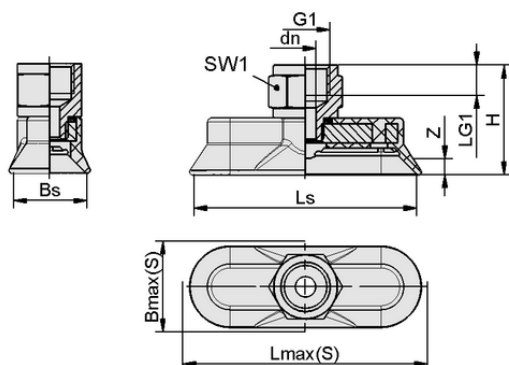
デザインデータ SAOG 60x20 NBR-45 G3/8-IG
