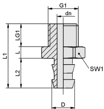
デザインデータ SA-NIP N035 G1/8-AG DN500
