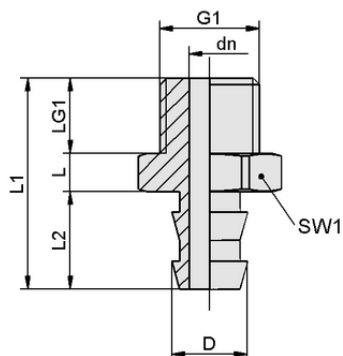
Конструктивные данные SA-NIP N035 G1/8-AG DN500
