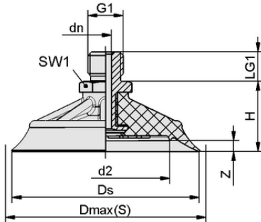
Tasarım verileri SHFN 50 NK-45 G1/4-AG MOS-TV
