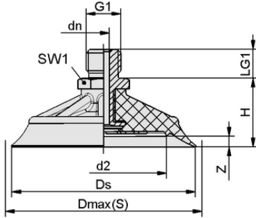
Tasarım verileri SHFN 70 NK-45 G1/4-AG MOS-TV
