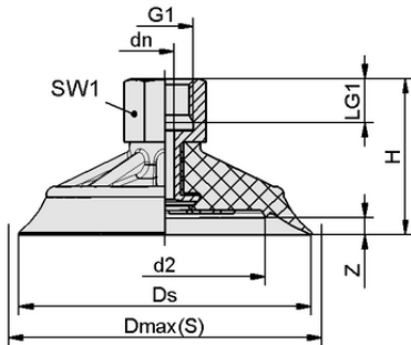
Tasarım verileri SHFN 50 NK-45 G1/4-IG
