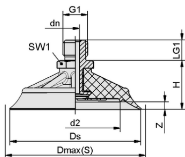
Конструктивные данные SHFN 50 NK-45 G1/4-AG
