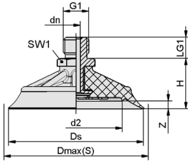
Tasarım verileri SHFN 70 NK-45 G1/4-AG MOS
