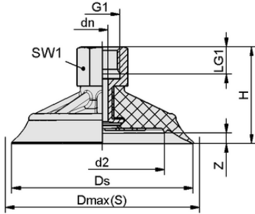
Tasarım verileri SHFN 70 NK-45 G1/4-IG
