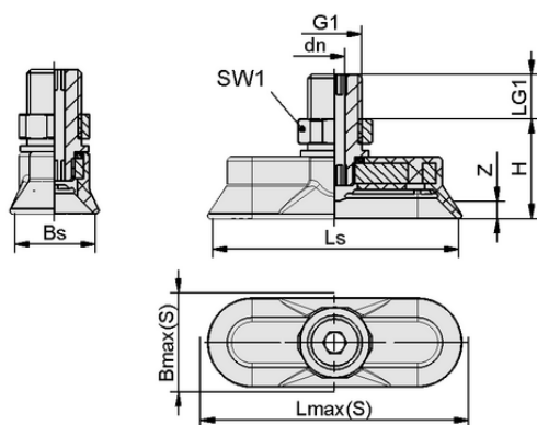
Données de construction SAOG 80x30 NBR-45 G1/4-AG
