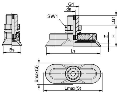
Конструктивные данные SAOG 80x30 NBR-45 G3/8-AG
