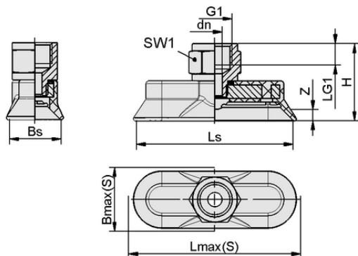
デザインデータ SAOG 80x30 NBR-45 G1/4-IG
