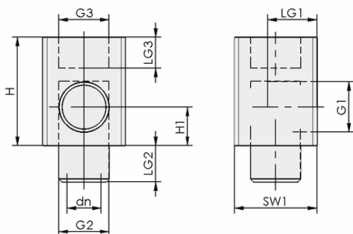
Конструктивные данные ANW G3/8-IG G3/8-AG
