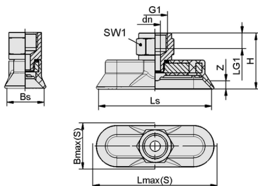
デザインデータ SAOG 80x30 NBR-45 G3/8-IG
