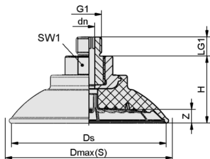
Конструктивные данные SAF 80 NBR-45 G3/8-AG
