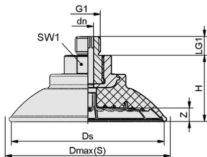
Конструктивные данные SAF 60 NBR-45 G1/4-AG
