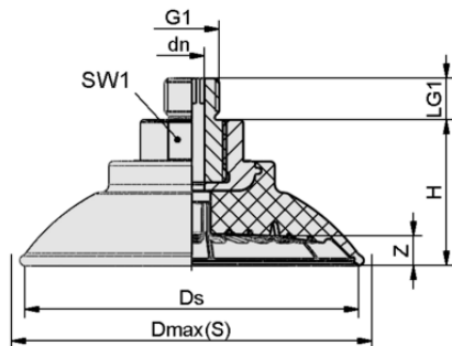
Datos de diseño SAF 60 NBR-45 G3/8-AG
