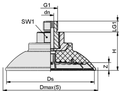
Конструктивные данные SAF 40 NBR-45 G3/8-AG
