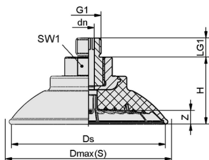
Конструктивные данные SAF 30 NBR-45 G1/4-AG
