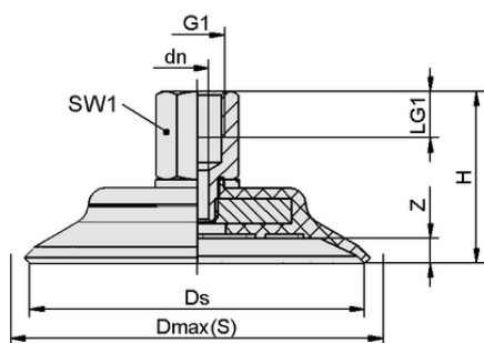
Конструктивные данные PFYN 80 HT1-60 G1/4-IG
