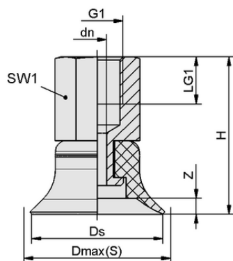
Design data PFYN 15 HT1-60 G1/8-IG
