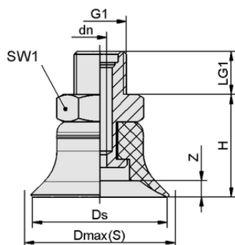
Конструктивные данные PFYN 35 HT1-60 G1/8-AG
