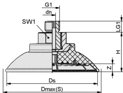
デザインデータ SAF 100 NBR-60 G3/8-AG
