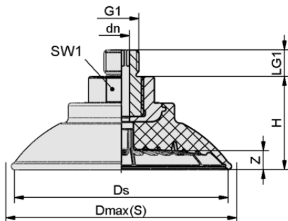
Dati di costruzione SAF 80 NBR-60 G3/8-AG
