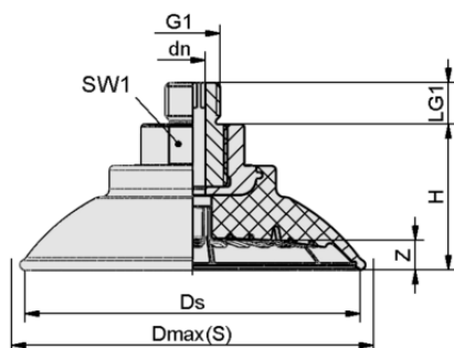
Конструктивные данные SAF 80 NBR-60 G3/8-AG
