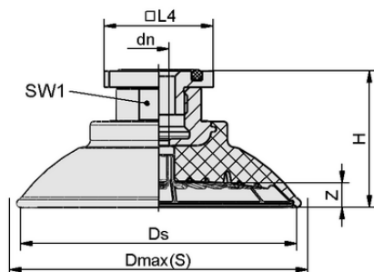
Données de construction SAF 100 NBR-60 RA
