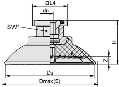
Tasarım verileri SAF 100 NBR-60 RA
