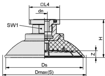
Données de construction SAF 80 NBR-60 RA
