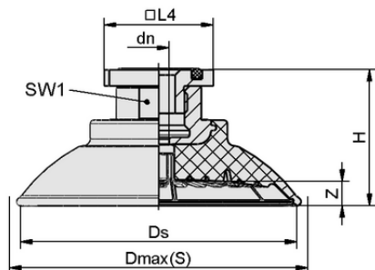
Конструктивные данные SAF 80 NBR-60 RA
