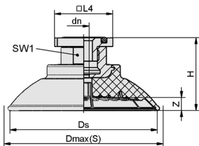
Dati di costruzione SAF 60 NBR-60 RA
